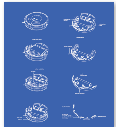
Éclaté de Robot aspirateur
